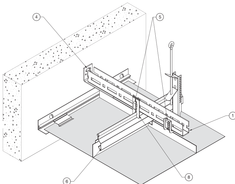
Rysunek systemu (moduł 600 x 600mm)
